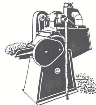
Kombinerad redningsmaskin för maskinkraft med dammsugning
