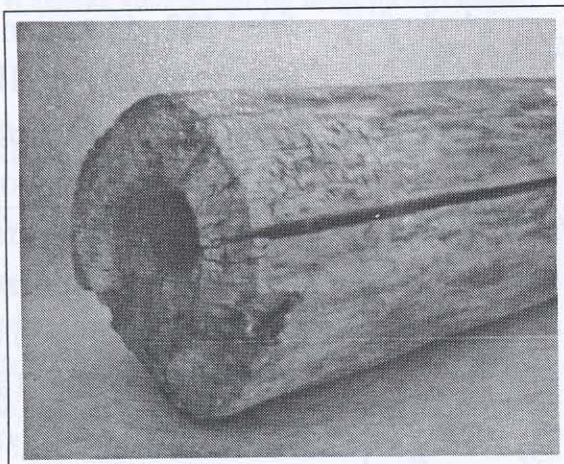
Änden av en vattenledningsstock, där man ser hur själva hålet borrats i stockens mitt.
